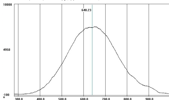
ハロゲンランプ放射スペクトル
